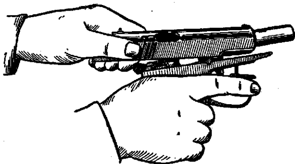
Рис. 5. Отделение затвора от рамки
