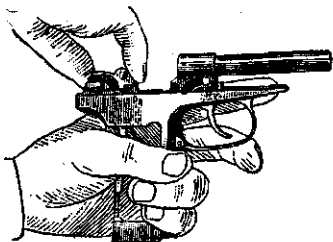
Рис. 13. Отделение курка от рамки
