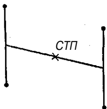
Рис. 50. Определение средней точки попадания по четырем симметрично расположенным пробойнам
