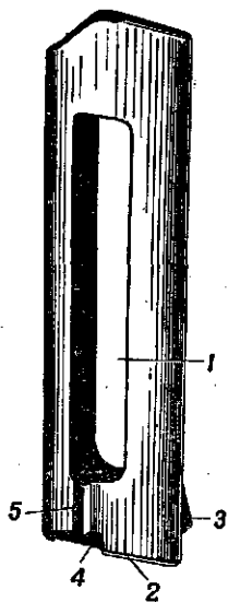
Рис. 40. Корпус мага- зина: 1 — окно; 2 — загнутое реб- ро; 3 — выступ; 4 — вырез; 5 — желоб
