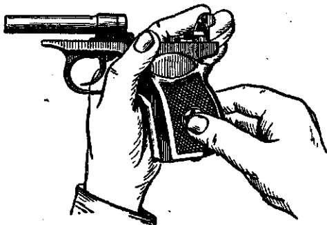
Рис. П. Отделение рукоятки от основания рукоятки
