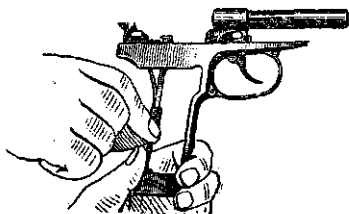
Рис. 23. Закрепление боевой пружины задвижкой
