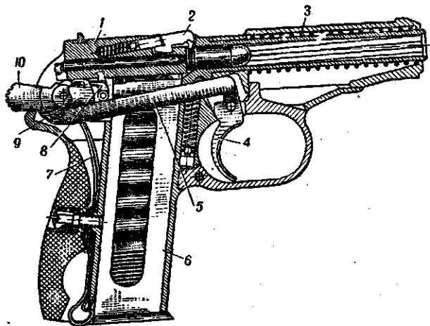
Рис. 46. Положение частей и механизмов пистолета перед выстрелом:
