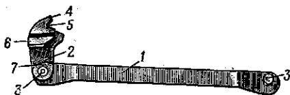
Рис. 34. Спусковая тяга с рычагом взвода: 1 — спусковая тяга; 2 — рычаг взвода; 3 — цапфы спусковой тяги; 4 — разобщающий выступ рычага взвода; 5 — вырез; 6 — выступ самовзвода; 7 — пяточка рычага взвода
