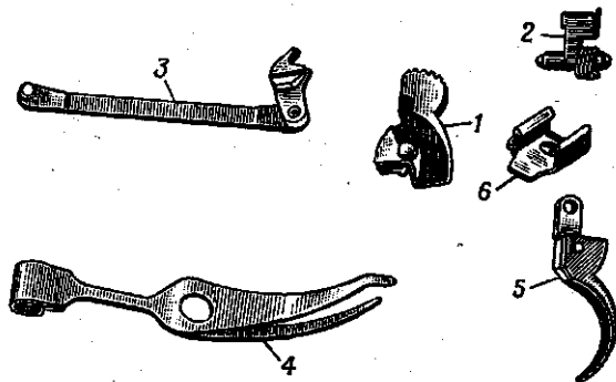
Рис. 31. Части ударно-спускового механизма:
