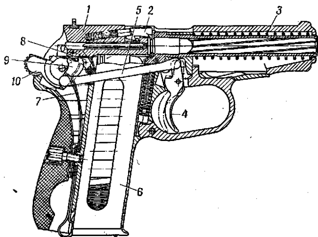
Рис. 47. Положение частей и механизмов пистолета перед выстрелом самовзводом:
