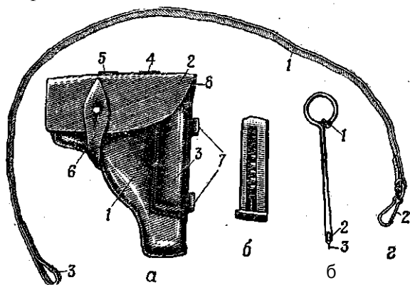
Рис. 44. Принадлежность к пистолету:
