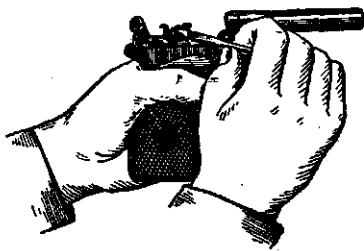
Рис. 9. Снятие крючка пружины шептала с затворной задержки
