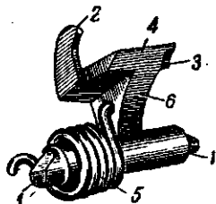
Рис. 33. Шептало: 1 — цапфы шептала; 2 — зуб; 3 — выступ; 4 — носик шептала; 5 — пружина шептала; 6 — стойка шептала
