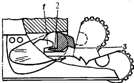
Рис. 48. Схема блокировки курка выступом предохранителя:
